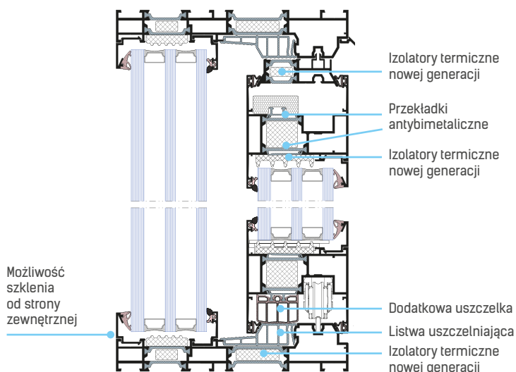
Przekrój pionowy – rama ze szkleniem stałym
