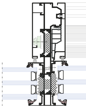
Połączenie AS 75 z AS 178HS
