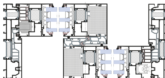
Przekrój poziomy
