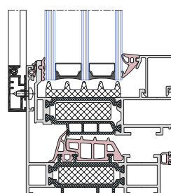
Moskitiera ramkowa przykręcana
