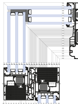
Naroże całoszklane w systemie AS 178HS
